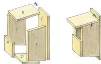
Modèle de nichoir boîte à lettres
